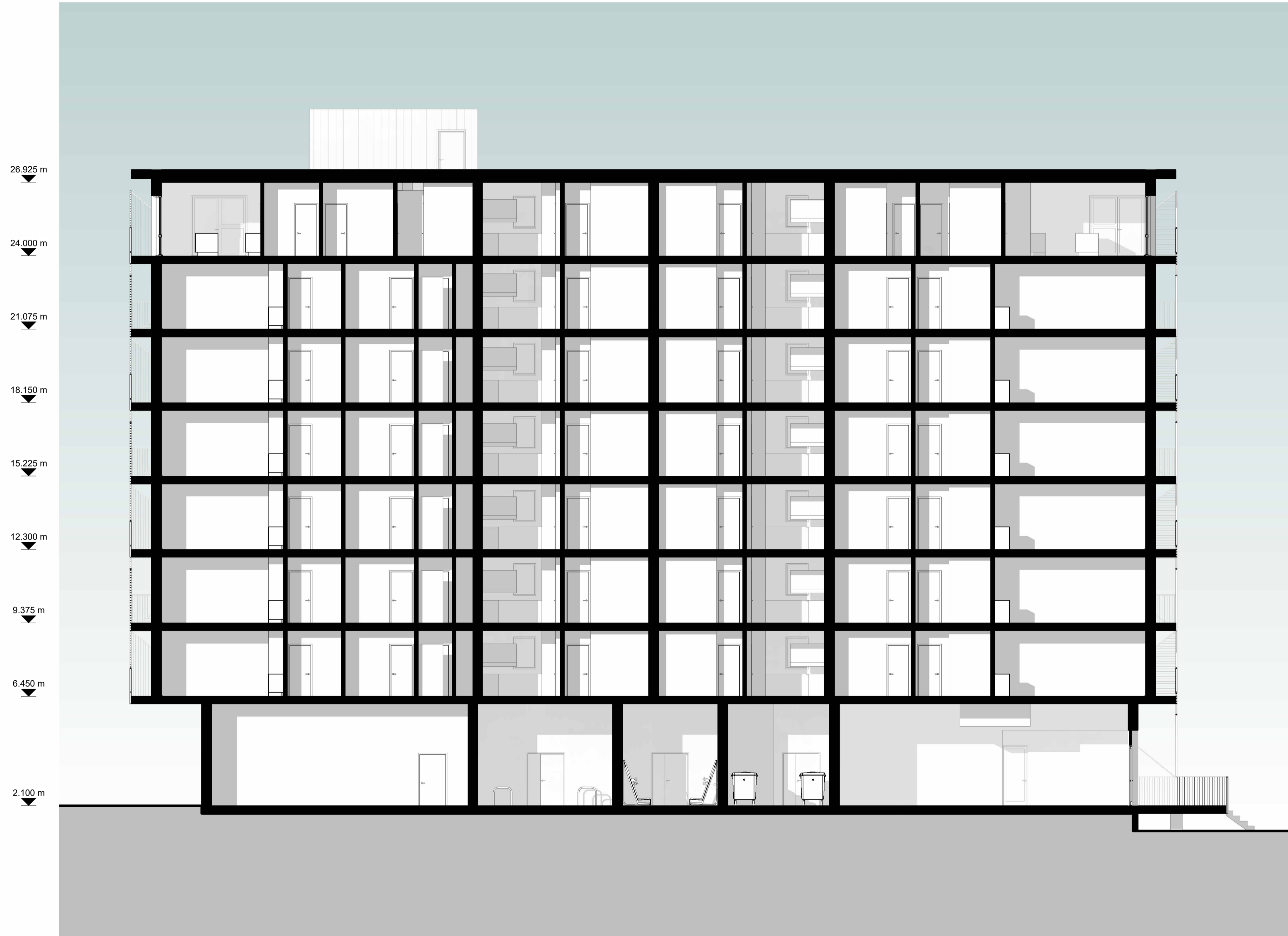
2 Section 2 1 : 100
