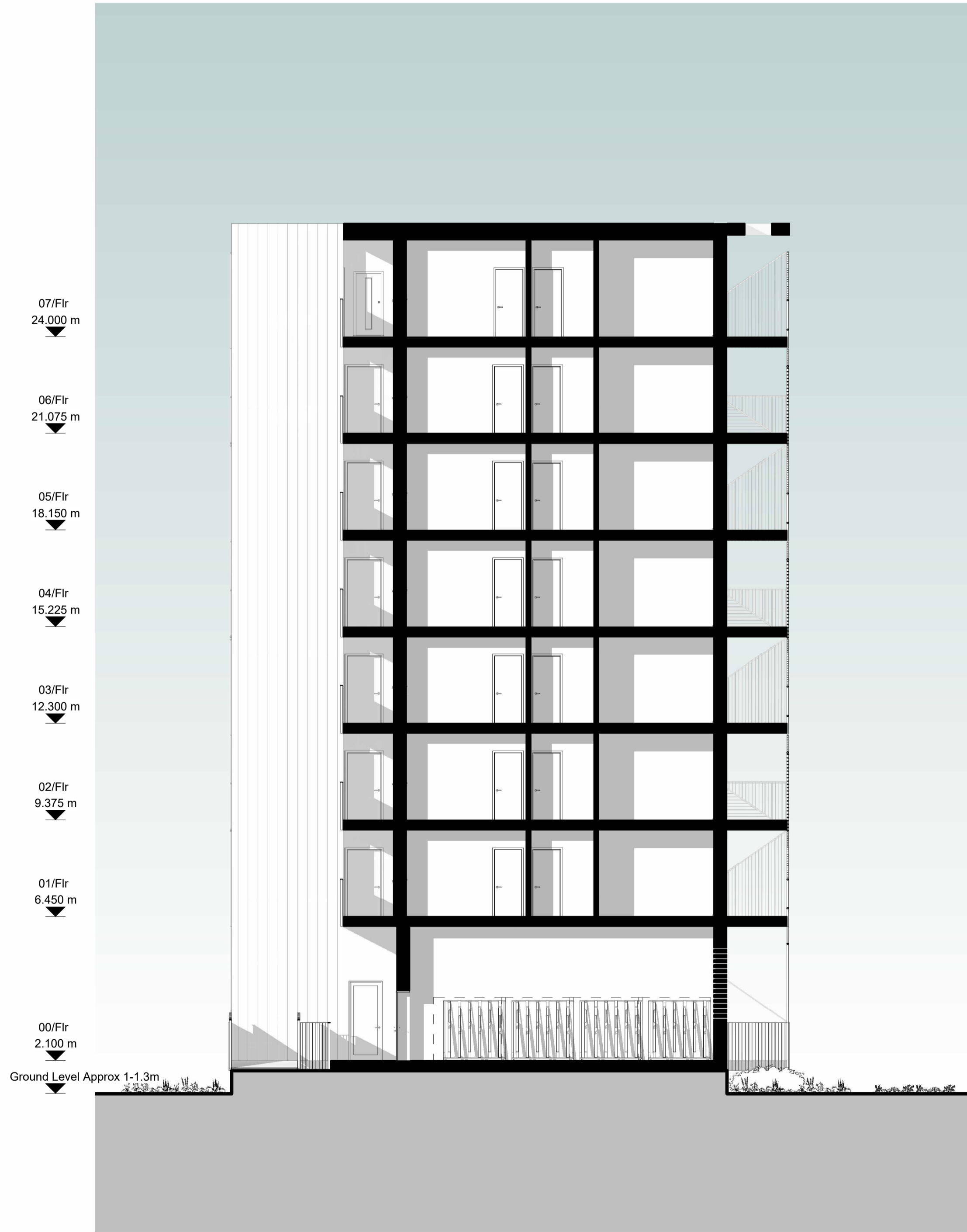
1 Section 1 1 : 100
