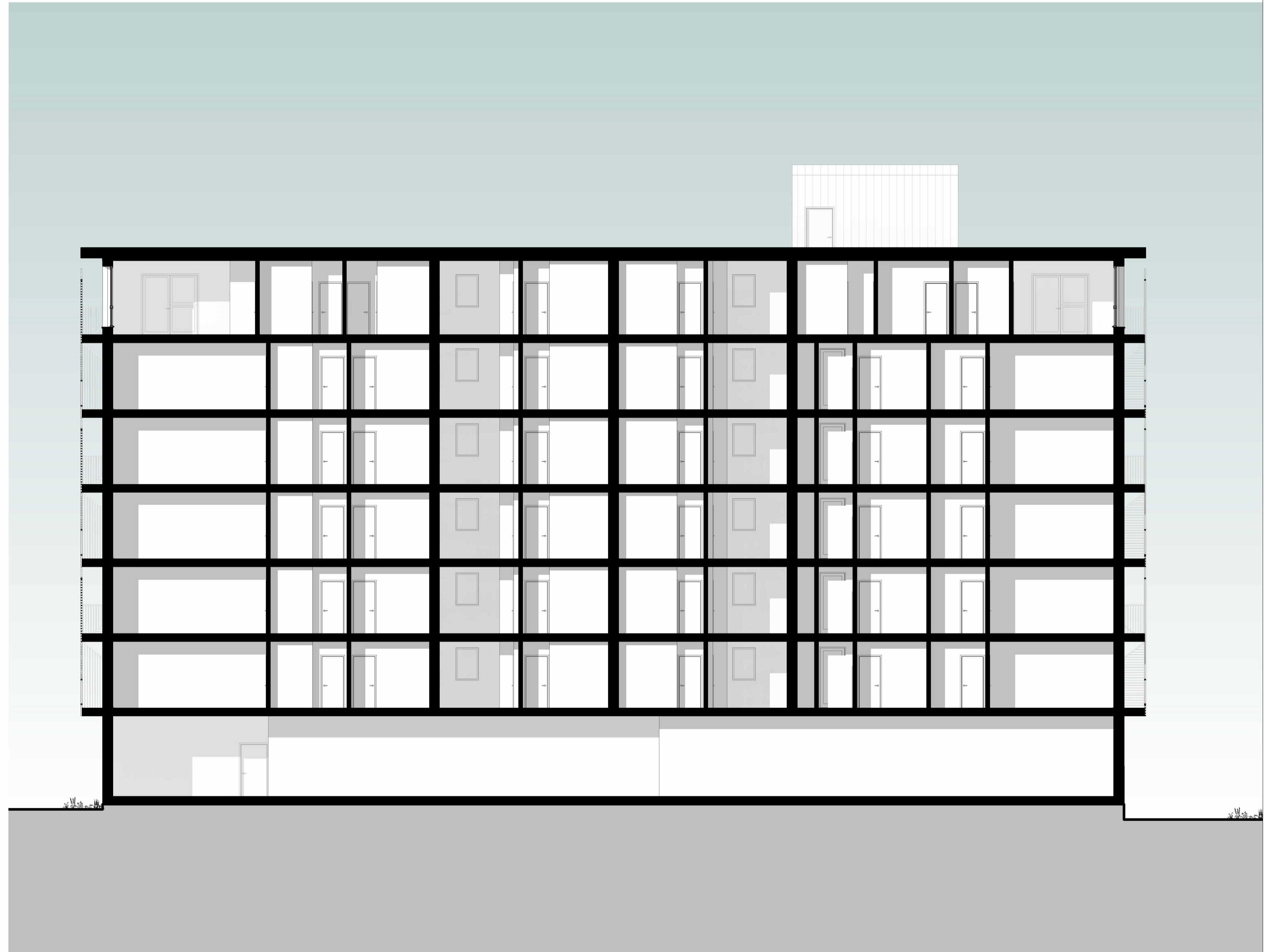
2 Section 2 1 : 100
