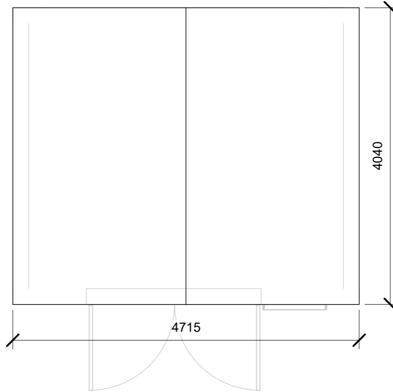
2 01/Flr 1:50
