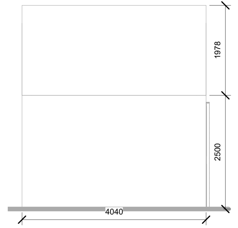
4 Side Elevation 1:50
