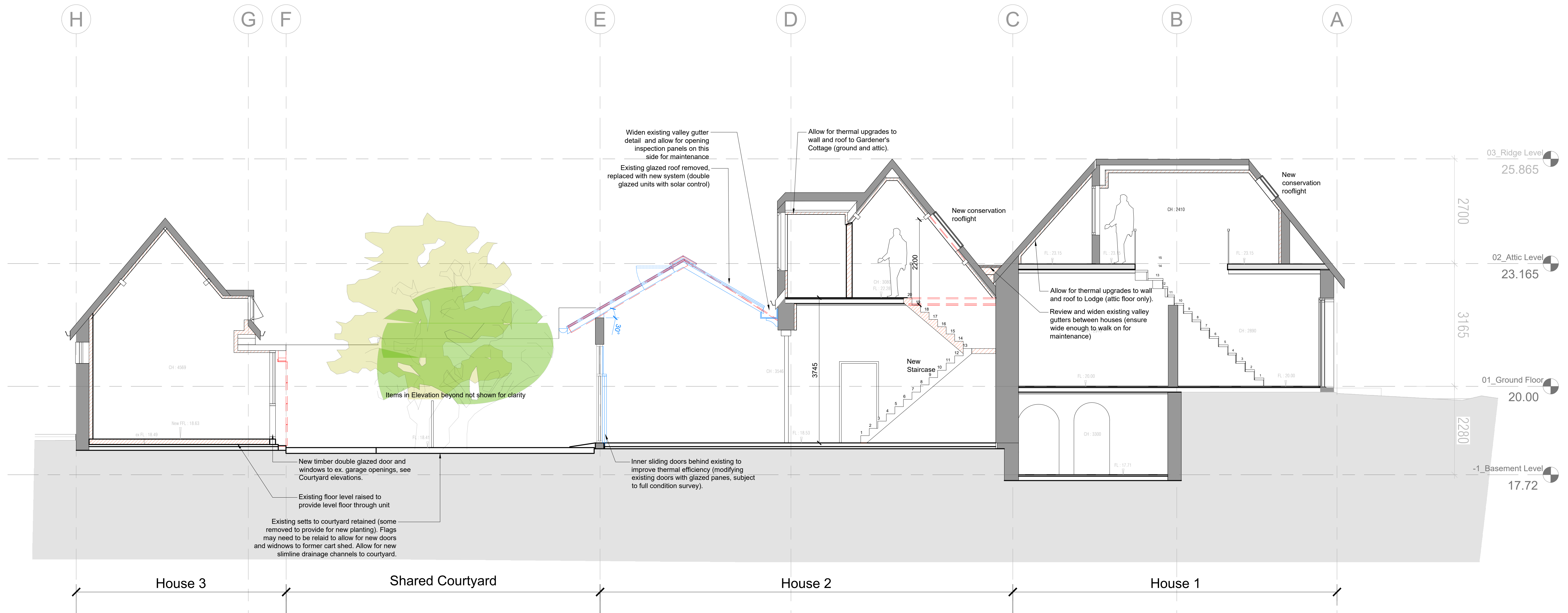
1 Section 01 2150 1:50
